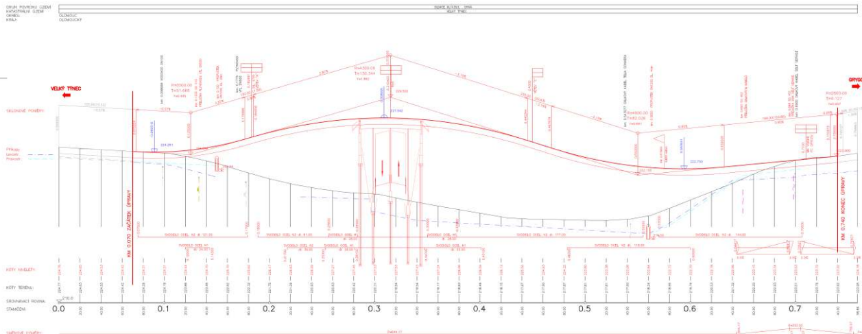
PODÉLNÝ PROFIL M 1 : 1000/100
