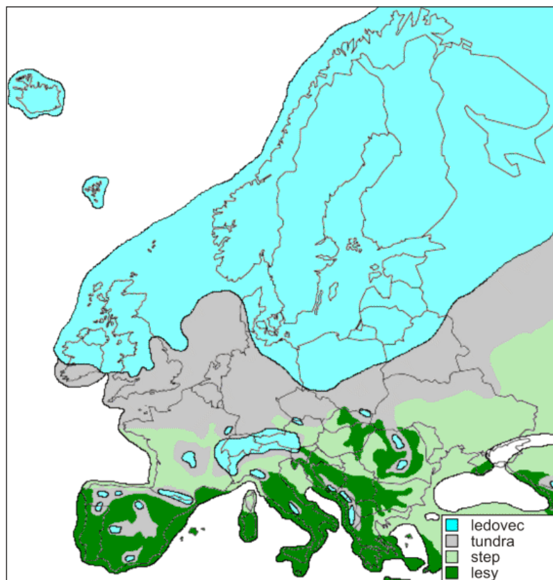
Rozsah kontinentálního ledovce v Evropě v období před 20 tisíci lety. Zdroj: www.geocities.com
